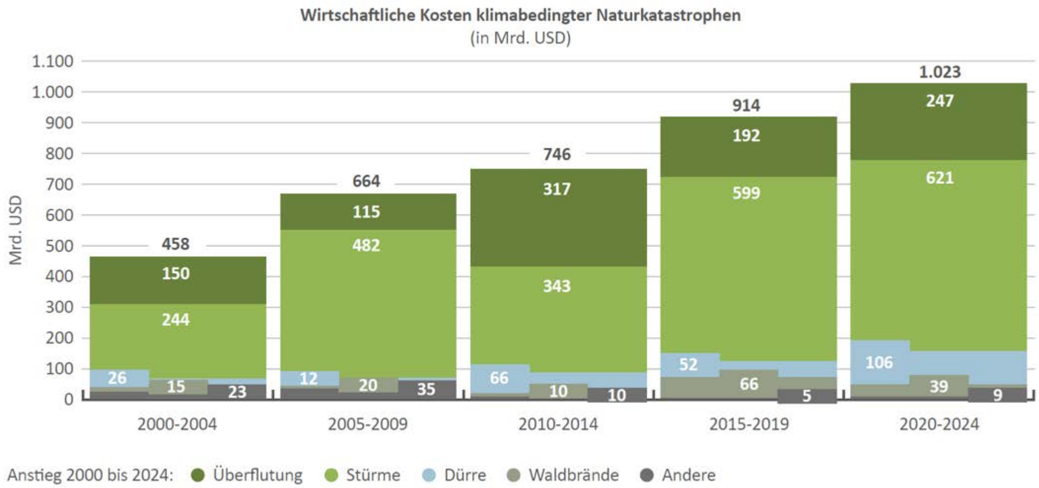
Abb. 4: Weltweit steigende Kosten von Naturkatastrophen und Extremwetterereignissen
