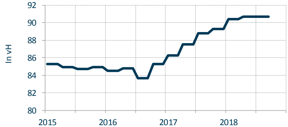
Maschinenbau: Kapazitätsauslastung
