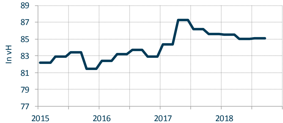
Chemie: Kapazitätsauslastung
